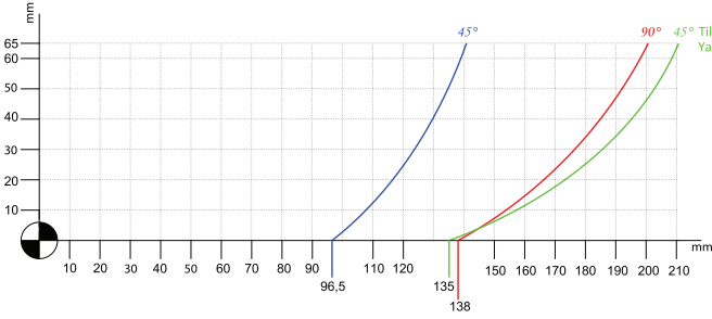
Alya Ø305 mm
