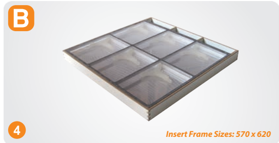
Alüminyum Teloralı B Tipi Kasa B Type Sieve Box With Aluminum Insert Frame
