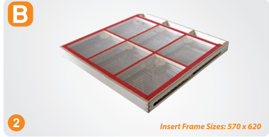
Ahşap Teloralı B Tipi Kasa B Type Sieve Box With Wooden Insert Frame
