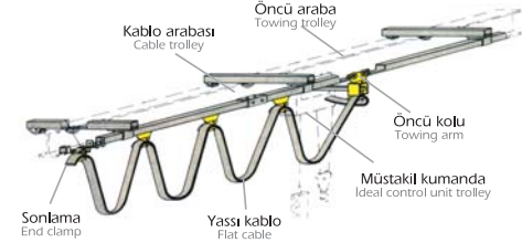
Vinç Kablo Taşıma Sistemi Crane Festoon System
