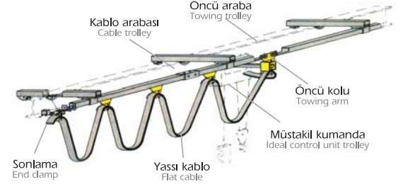
Vinç Kablo Taşıma Sistemi Crane Festoon System
